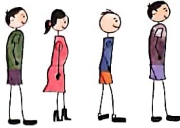
queue
